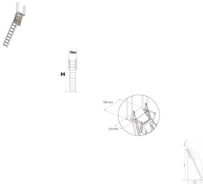
Escalera Escamoteable de tijera para altillos
